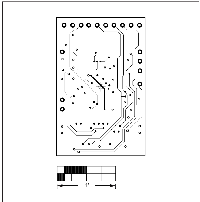
MAX86141OSBEK#—L03 SIG
