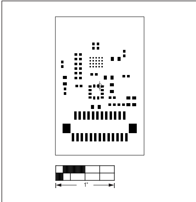
MAX86141OSBEK#—Top Paste
