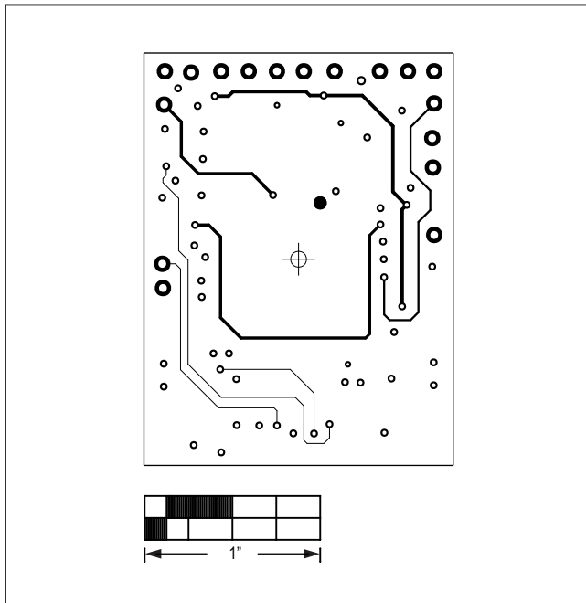
MAX86140SBEK#—L04 SIG
