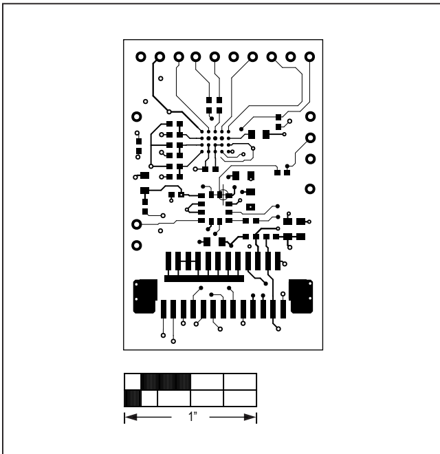
MAX86141OSBEK#—Top
