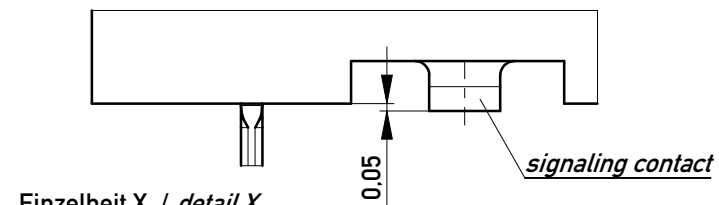
Einzelheit X / detail X M 20:1 / scale 20:1
