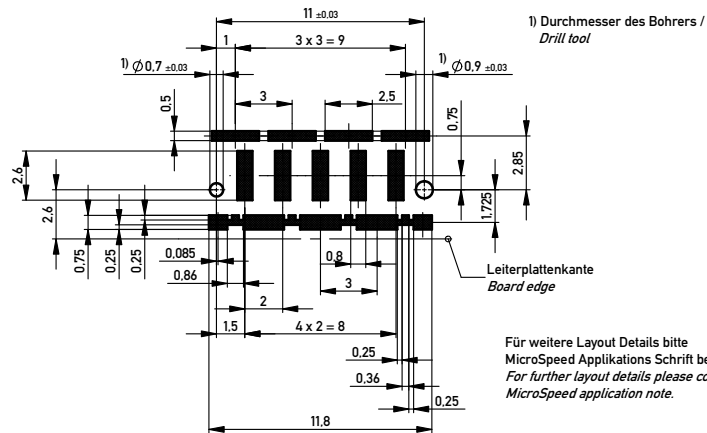
Leiterplatten-Layout Vorschlag / PCB-layout proposal
