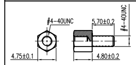
4.8*10.5 SCREW
