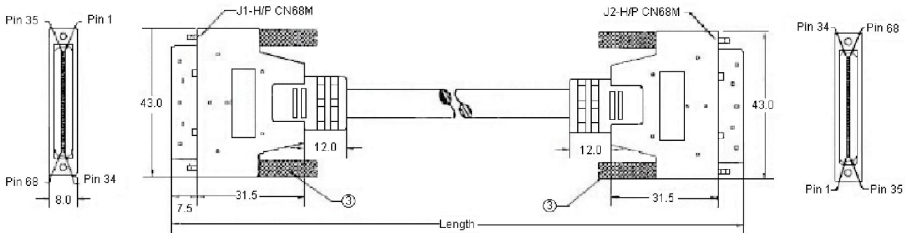
Dimensions : Millimetres
