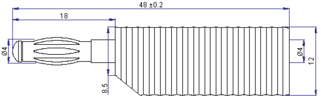
Dimensions : Millimetres
