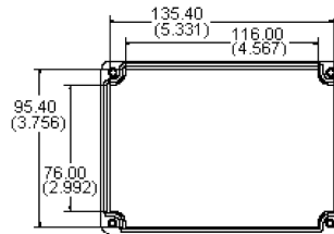
Lid - Inside
