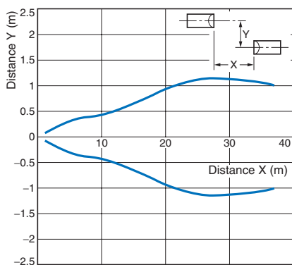
Diffuse-reflective E3S-CD□□ (-M1J)
