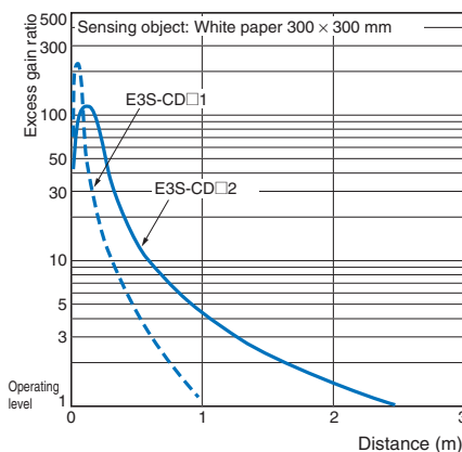
Diffuse-reflective E3S-CD□□ (-M1J)
