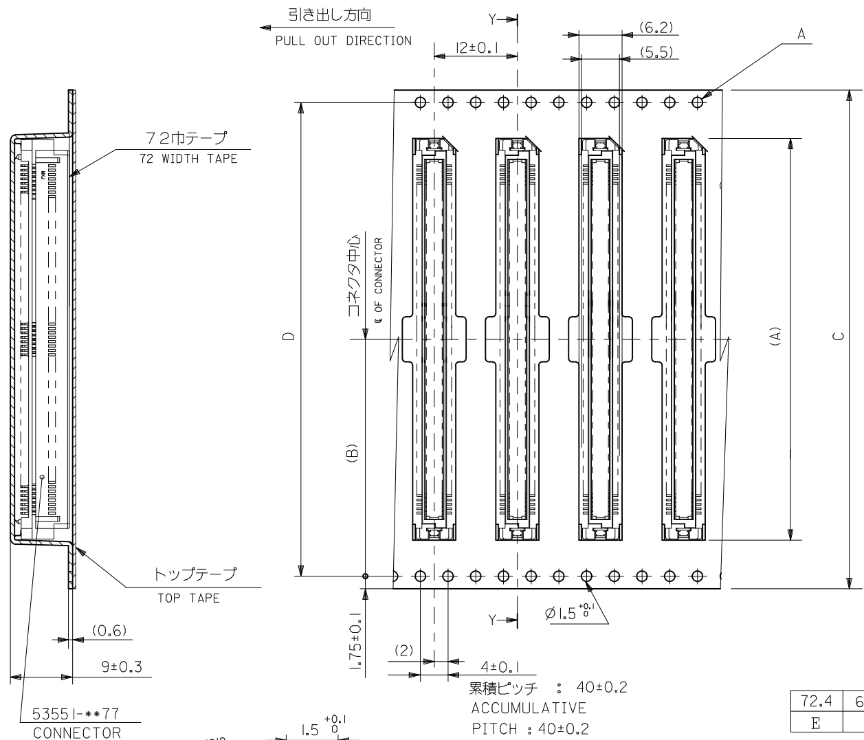
断面 Y-Y SECTION Y-Y
