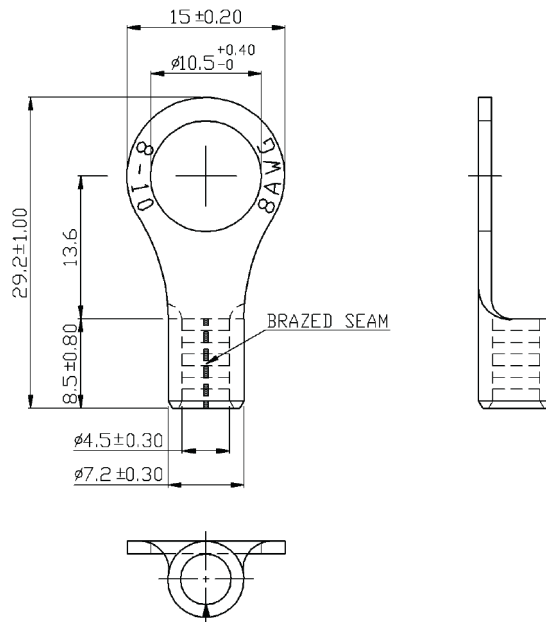
Dimensions : Millimeters
