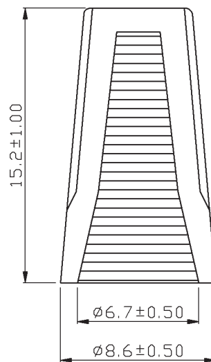
Dimensions : Millimetres
