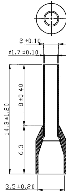
Dimensions : Millimetres
