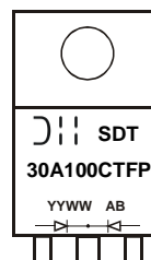
ITO220AB
