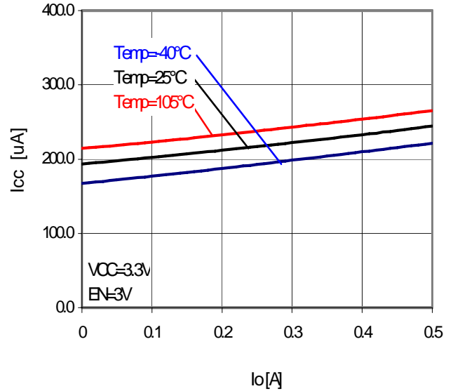
Fig.30 I_o-I_{CC}
