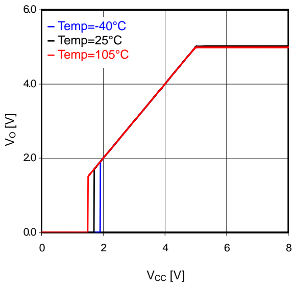
Fig. 27 V CC -V O (I O =0mA)
