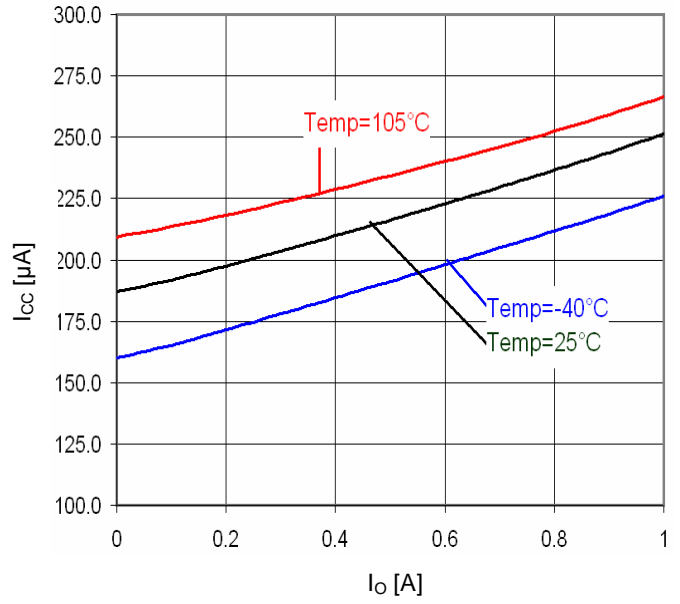
Fig.32 I o -I cc
