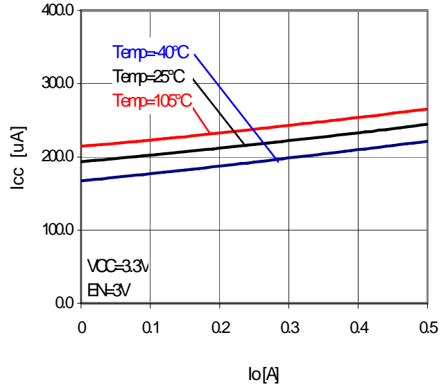
Fig.30 I_o-I_{cc}
