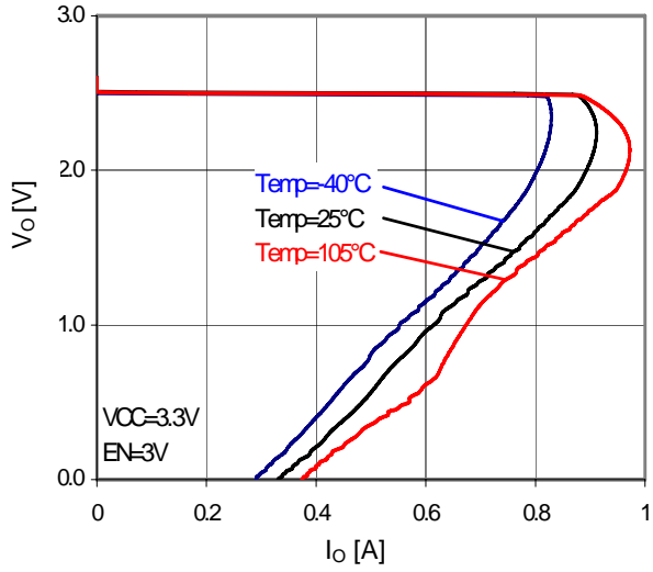
Fig.29 OCP
