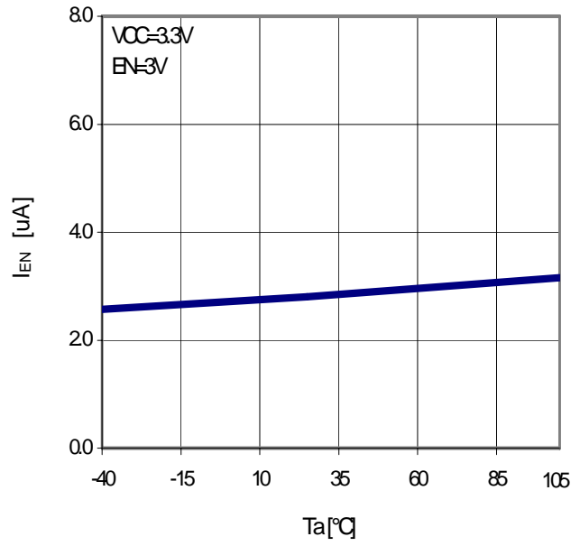
Fig.24 T_a - I_{EN}
