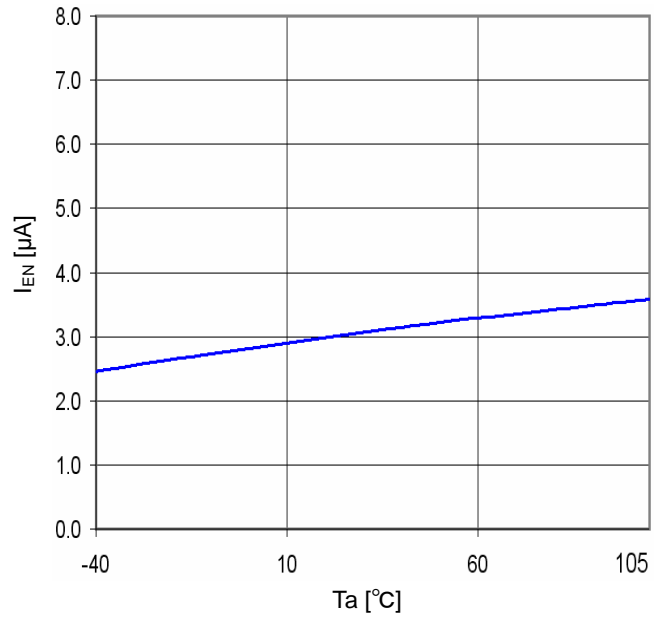
Fig.24 T_a - I_{EN}
