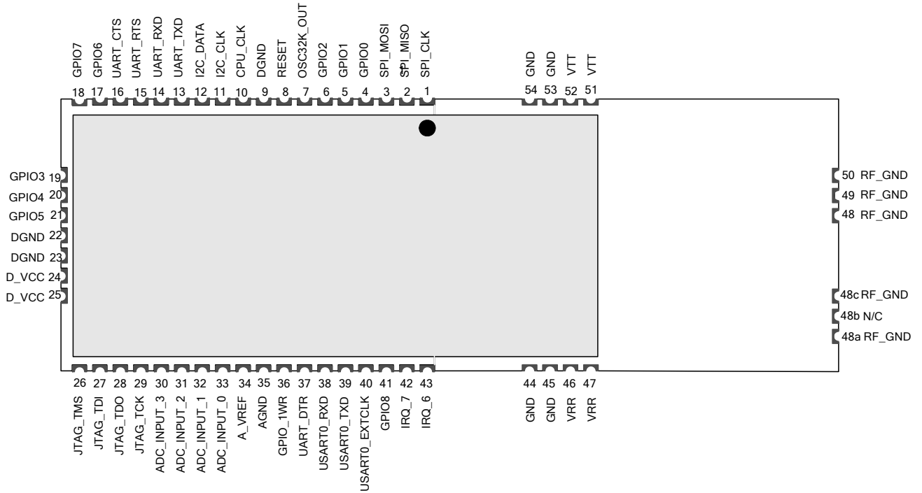
ZDM-A1281-PN0 Pinout
