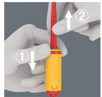
Durch Herunterziehen und Halten des Betätigungsschalters wird die Arretierung gelöst, und die Wechselklinge oder der Schaltschrankschlüssel kann entnommen werden.
