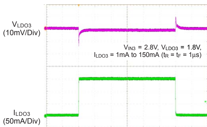
LDO3 Load Transient
