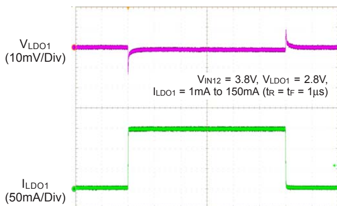
LDO1 Load Transient
