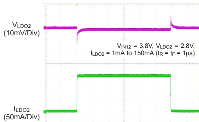
LDO2 Load Transient
