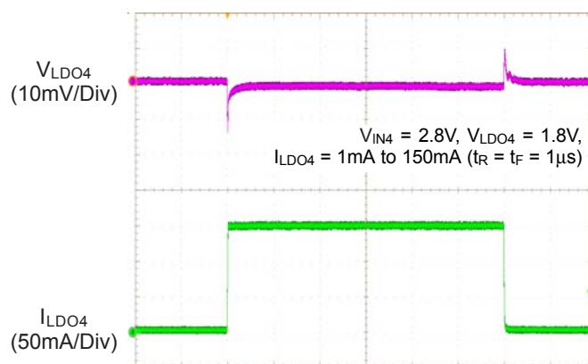
LDO4 Load Transient
