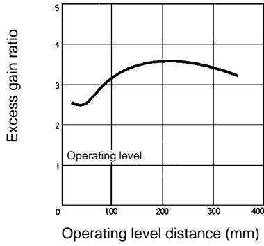
E3S-R11/-R61/-R16/-R66/-R31/-R81/-R36/-R86 with E39-R1
