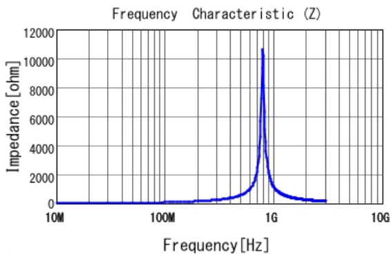
■ LQG15HSR12H02 |Z|
