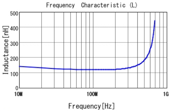
■ LQG15HSR12H02 L
