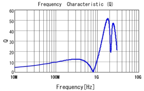
■ LQG15HSR12H02 Q
