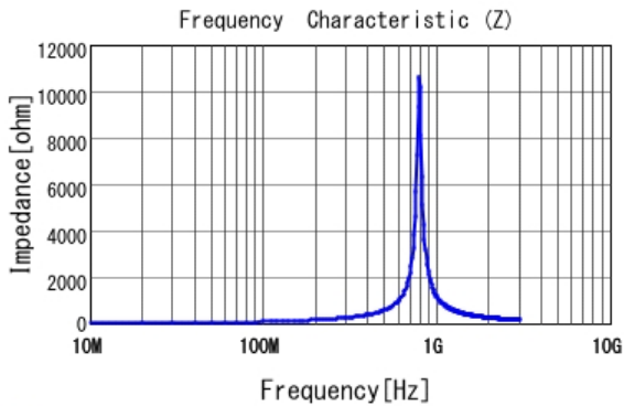
■ LQG15HSR12J02 |Z|
