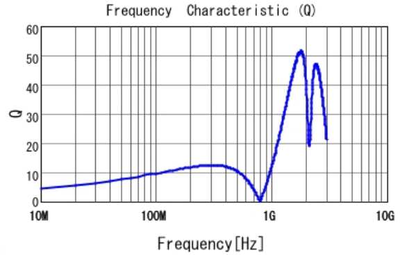
■ LQG15HSR12J02 Q
