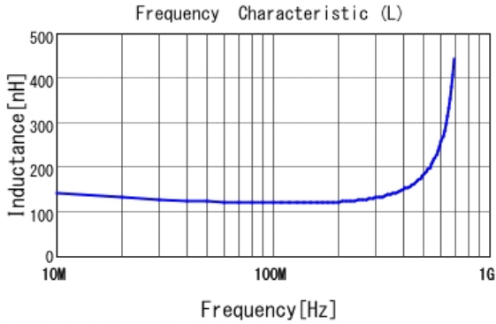
■ LQG15HSR12J02 L
