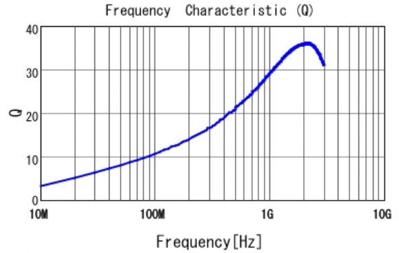
■ LQG15HZ6N8J02 Q
