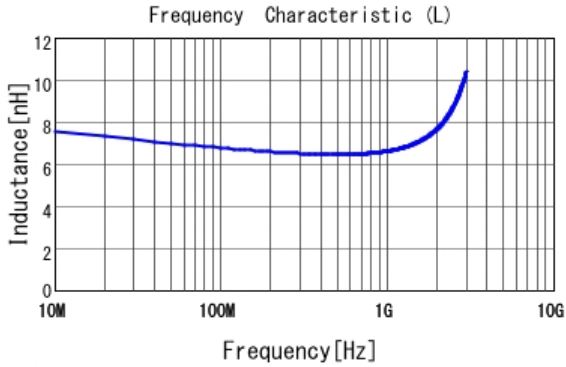
■ LQG15HZ6N8J02 L
