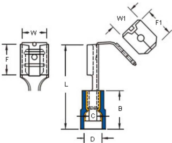
Dimensions : Inches (Millimetres)
