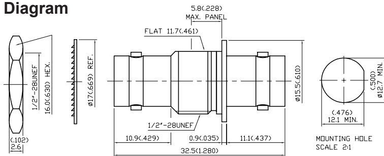
Dimensions : Millimetres (Inches)
