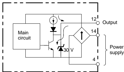
E3C-GE4 NPN Output Type
