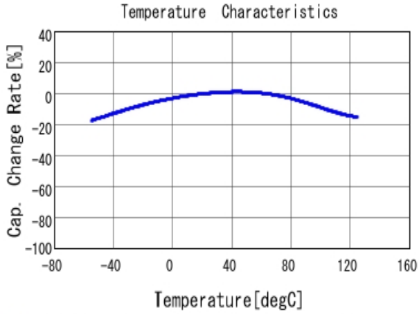
■ GRJ188C70J475KE11 C-Temp. capchange, DCO. 0V, ACO. 2V rm
