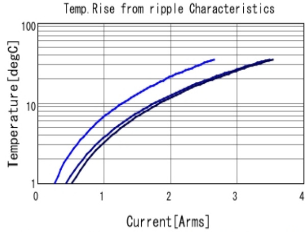
GRJ188C70J475KE11 Temp. rise ■ 100kHz ■ 500kHz ■ 1MHz
