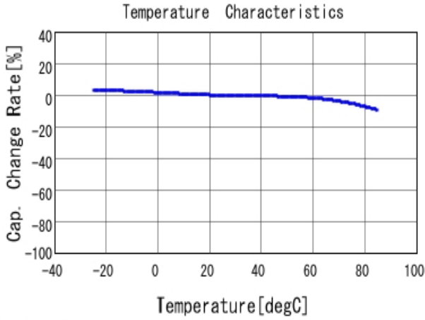
■ GRM188B31A106ME69 C-Temp. capchange, DCO. 0V, ACO. 5V rm
