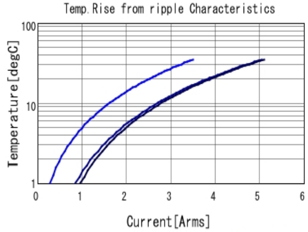
GRM188B31A106ME69 Temp. rise ■ 80kHz ■ 400kHz ■ 800kHz
