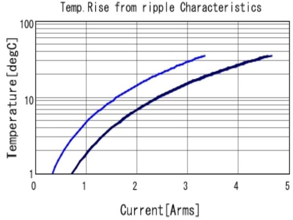
GRM319R61H475KA12 Temp. rise ■ 100kHz ■ 500kHz ■ 1MHz
