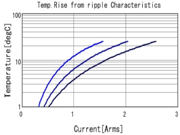
KRM31KR72A225KH01 Temp. rise ■ 50kHz ■ 100kHz ■ 300kHz
