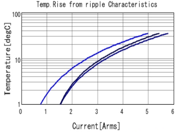
GRM188B30J226MEA0 Temp. rise ■ 80kHz ■ 400kHz ■ 800kHz
