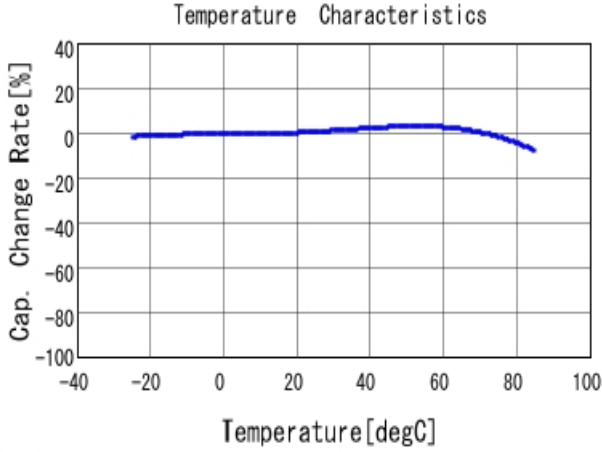
■ GRM188B30J226MEA0 C-Temp. capchange, DCO. 0V, ACO. 2V rm
