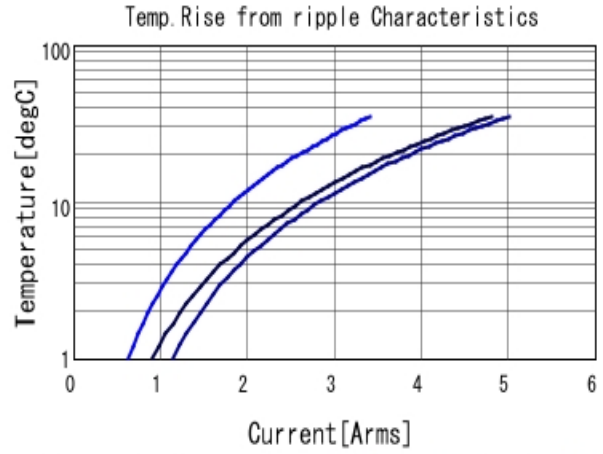
GRM188B31C475KAAJ Temp. rise ■ 100kHz ■ 500kHz ■ 1MHz
