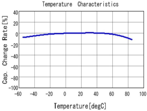
■ GRM319R61C226ME15 C-Temp. capchange, DCO. 0V, ACO. 5V rm
