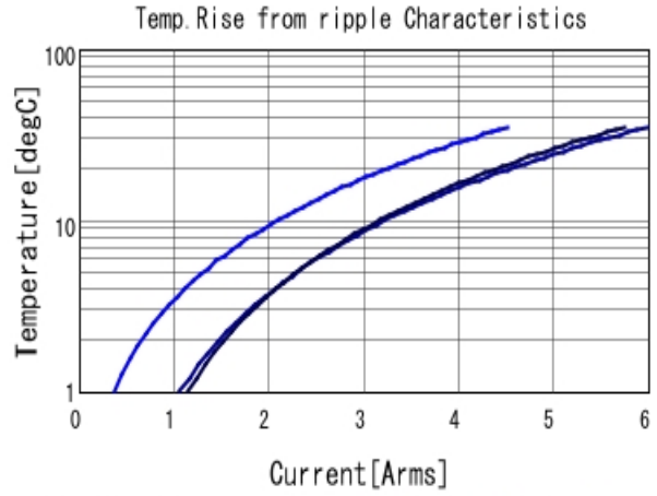
GRM319R61C226ME15 Temp. rise ■ 80kHz ■ 400kHz ■ 800kHz
