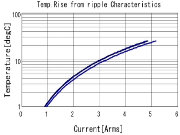
KRM55WR71E476MH01 Temp. rise ■ 50kHz ■ 100kHz ■ 300kHz
