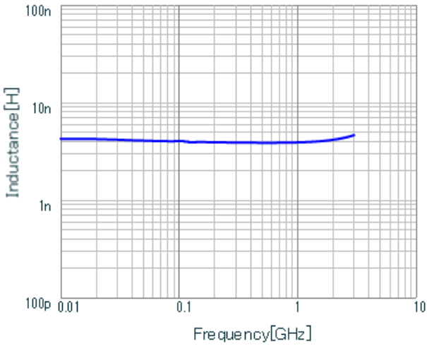
LQG15WZ4N1S02 L.
