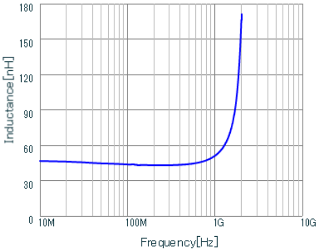
LQP03HQ43NJ02 L.
