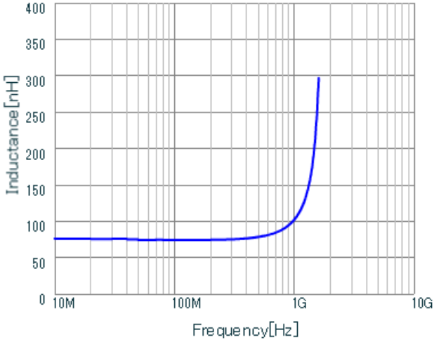
LQP03HQ75NJ02 L.
