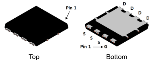
DFNW8 8.3x8.4, 2P CASE 507AP
