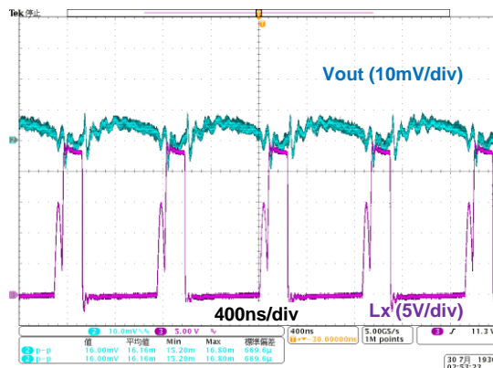
(4-4) Vin = 24V, Iout = 300mA
