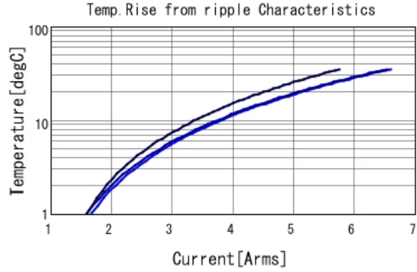
GCJ32EC71E226KE02 Temp. rise ■ 80kHz ■ 400kHz ■ 800kHz
