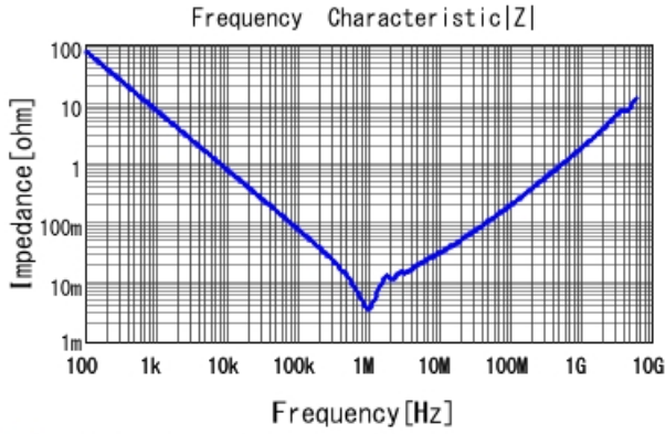
■ GCJ32EC71E226KE02 |Z| DC0V, 25degC
