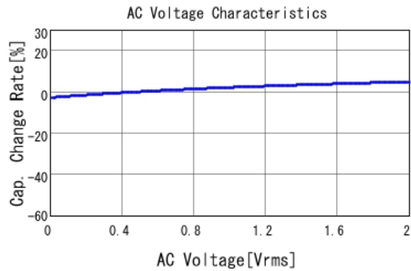
■ GCJ32EC71E226KE02 C-AC Voltage capchange, DC0V, 25.0d
