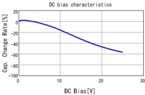
■ GCJ32EC71E226KE02 C-DC bias capchange, 25.0degC, AC0.
