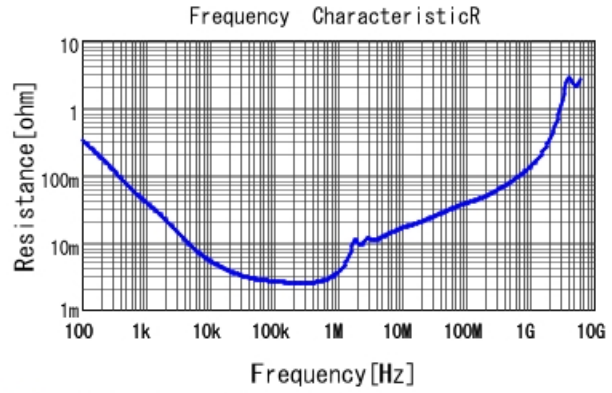
■ GCJ32EC71E226KE02 R DC0V, 25degC
