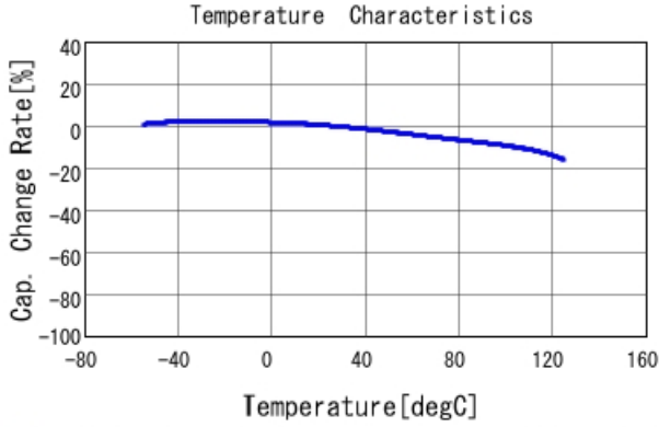
■ GCJ32EC71E226KE02 C-Temp. capchange, DCO. 0V, ACO. 5Vrm
