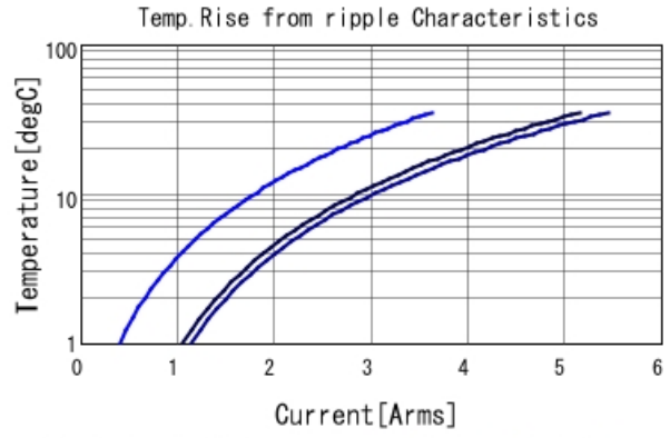
GRT31CC8YA106KE01 Temp. rise ■ 80kHz ■ 400kHz ■ 800kHz
