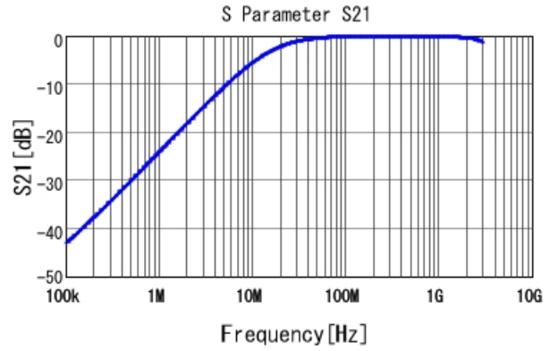
■ GA342QR7GD101KW01 S21 DCOV, 25degC
