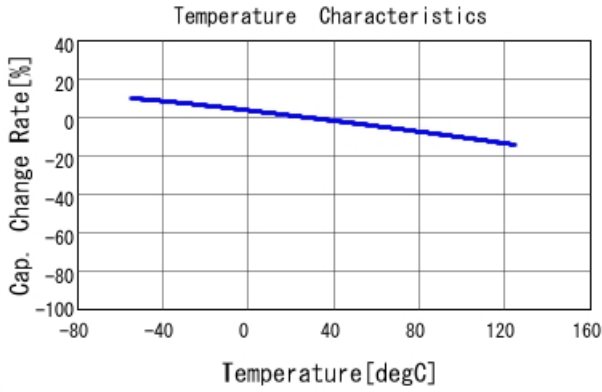
■ GA342QR7GD101KW01 C-Temp. capchange, DCOV, AC1Vrms
