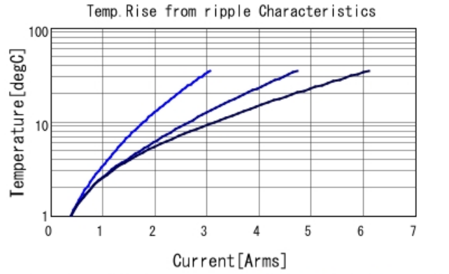
GC355XD72E105KX05 Temp. rise ■ 30kHz ■ 100kHz ■ 300kHz
