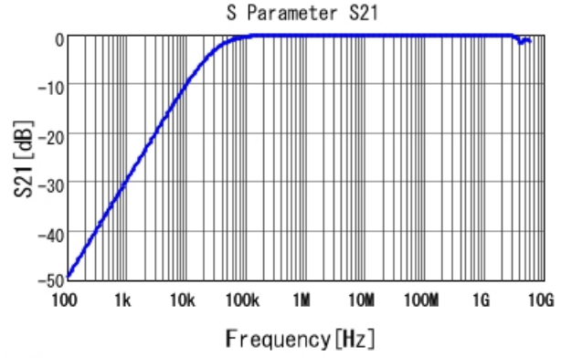
■ GCD21BR71H563KA01 S21 DCOV, 25degC
