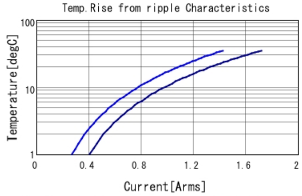
GCD21BR72A104KA01 Temp. rise ■ 500kHz ■ 1MHz
