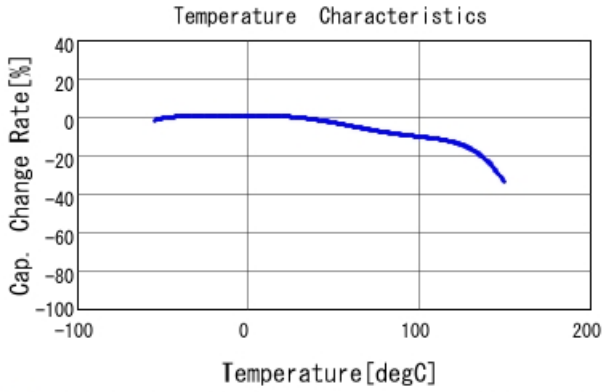
■ GCJ188L81E224KA01 C-Temp. capchange, DCO. 0V, AC1. 0Vrm
