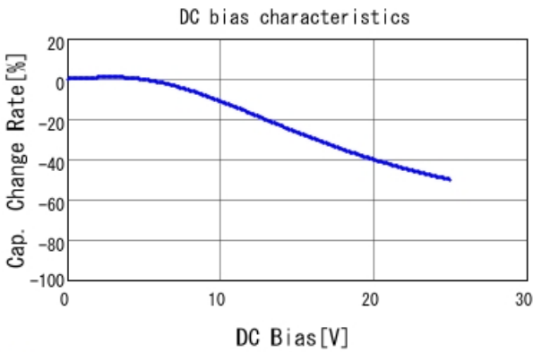
■ GCJ188L81E224KA01 C-DC bias capchange, 25.0degC, AC1.
