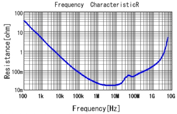
■ GCJ188L81E224KA01 R DC0V, 25degC
