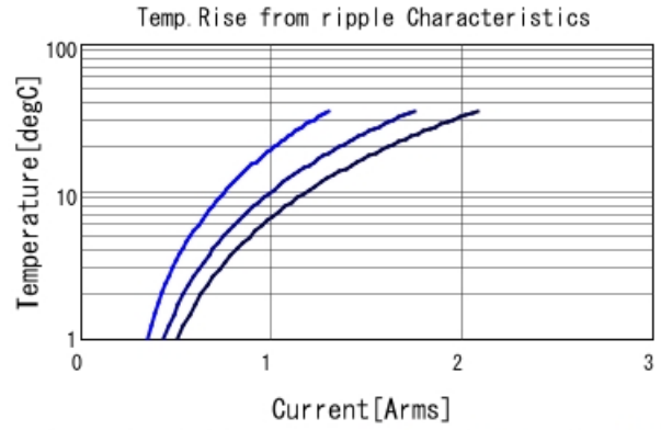
GCJ188L81E224KA01 Temp. rise ■ 300kHz ■ 600kHz ■ 1MHz
