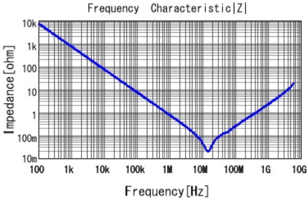
■ GCJ188L81E224KA01 |Z| DC0V, 25degC
