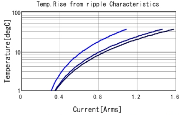
GCJ188R71A224KA01 Temp. rise ■ 300kHz ■ 600kHz ■ 1MHz
