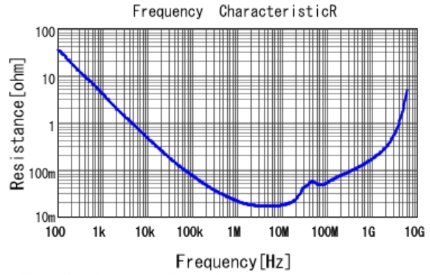
■ GCJ188R71A224KA01 R DC0V, 25degC
