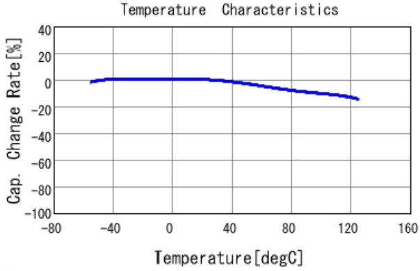
■ GCJ188R71A224KA01 C-Temp. capchange, DCO. 0V, AC1. 0Vrm
