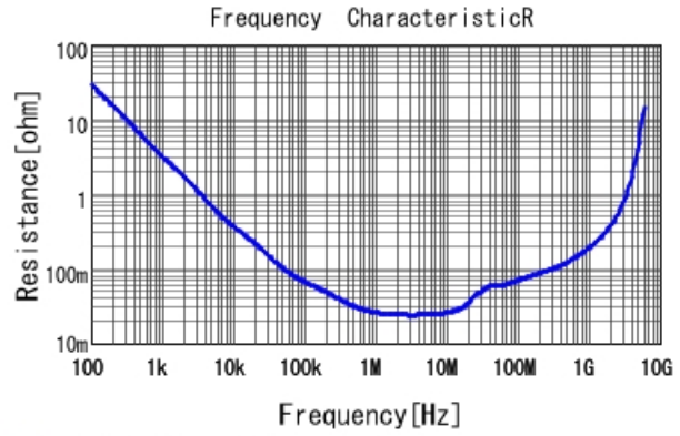
■ GCJ188R71C274KA01 R DC0V, 25degC
