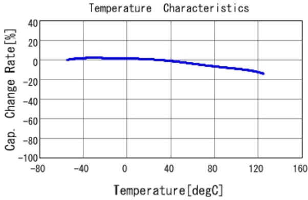
■ GCJ188R71C274KA01 C-Temp. capchange, DCO. 0V, AC1. 0Vrm
