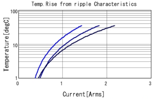
GCJ188R71C274KA01 Temp. rise ■ 300kHz ■ 600kHz ■ 1MHz
