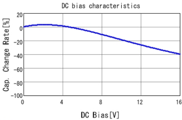
■ GCJ188R71C274KA01 C-DC bias capchange, 25.0degC, AC1.
