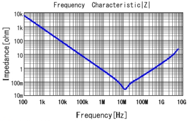
■ GCJ188R71C274KA01 |Z| DC0V, 25degC
